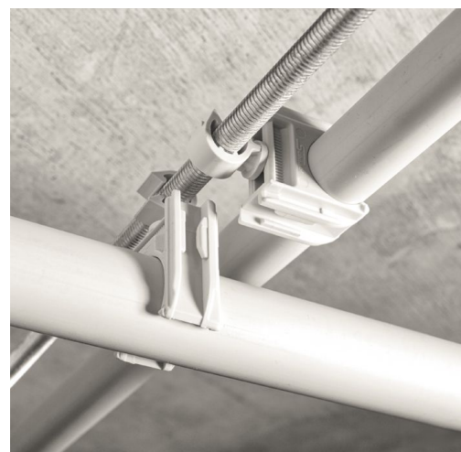
Mit dem SGC Schnabl Gewindeclip gelingt eine kraft- und zeitsparende Montage von Rohren auf Gewindestangen.
