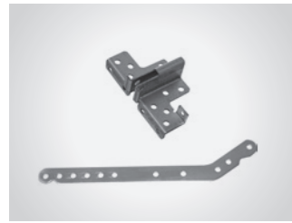
Torbeschlag Standard
