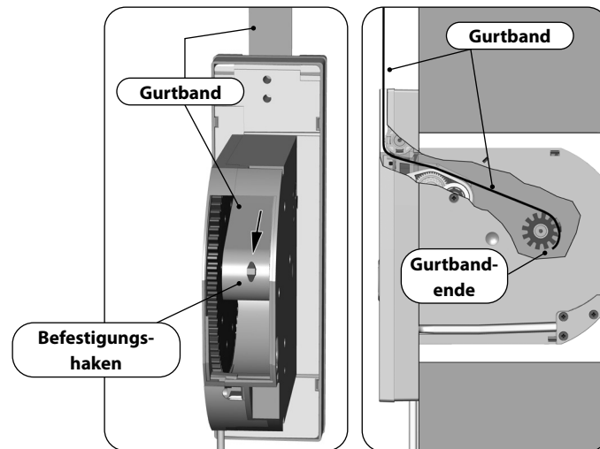
Gurtbandverlauf im Gurtwickler RolloTron classic smart
